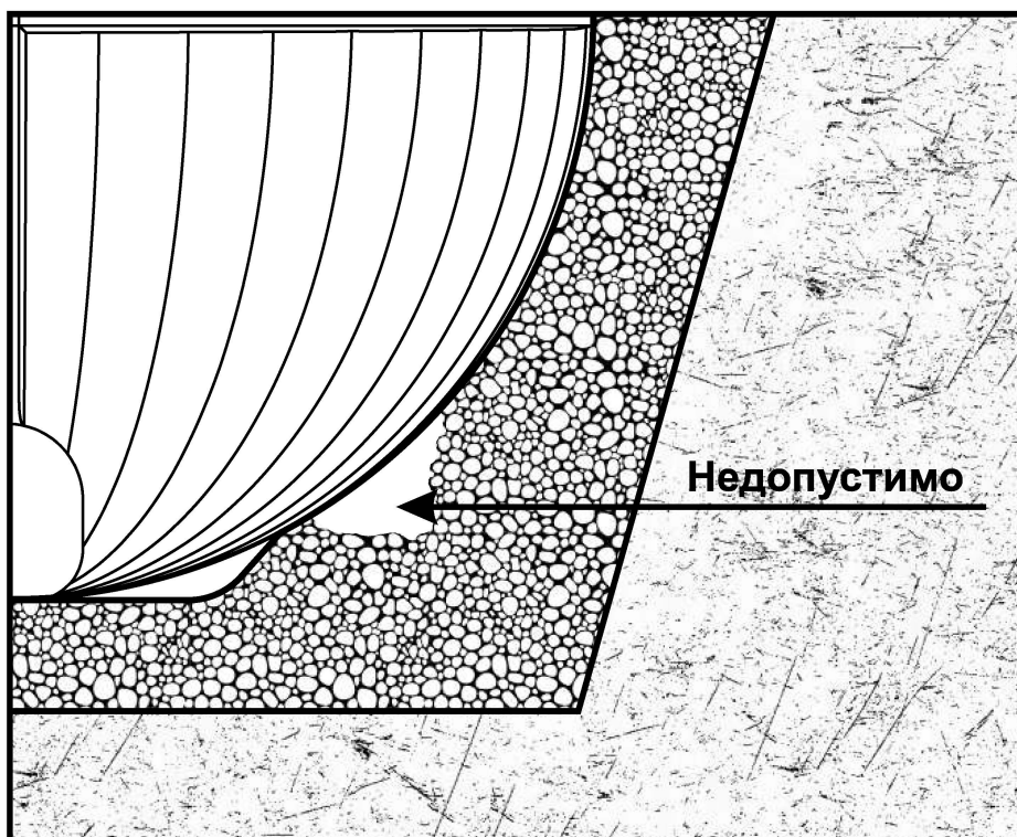
Рис 7. Обратная засыпка емкости
