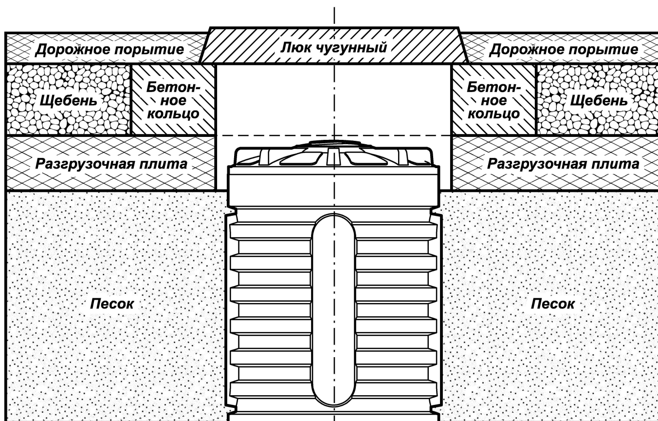
Рис 8. Монтаж емкости под проезжей частью
