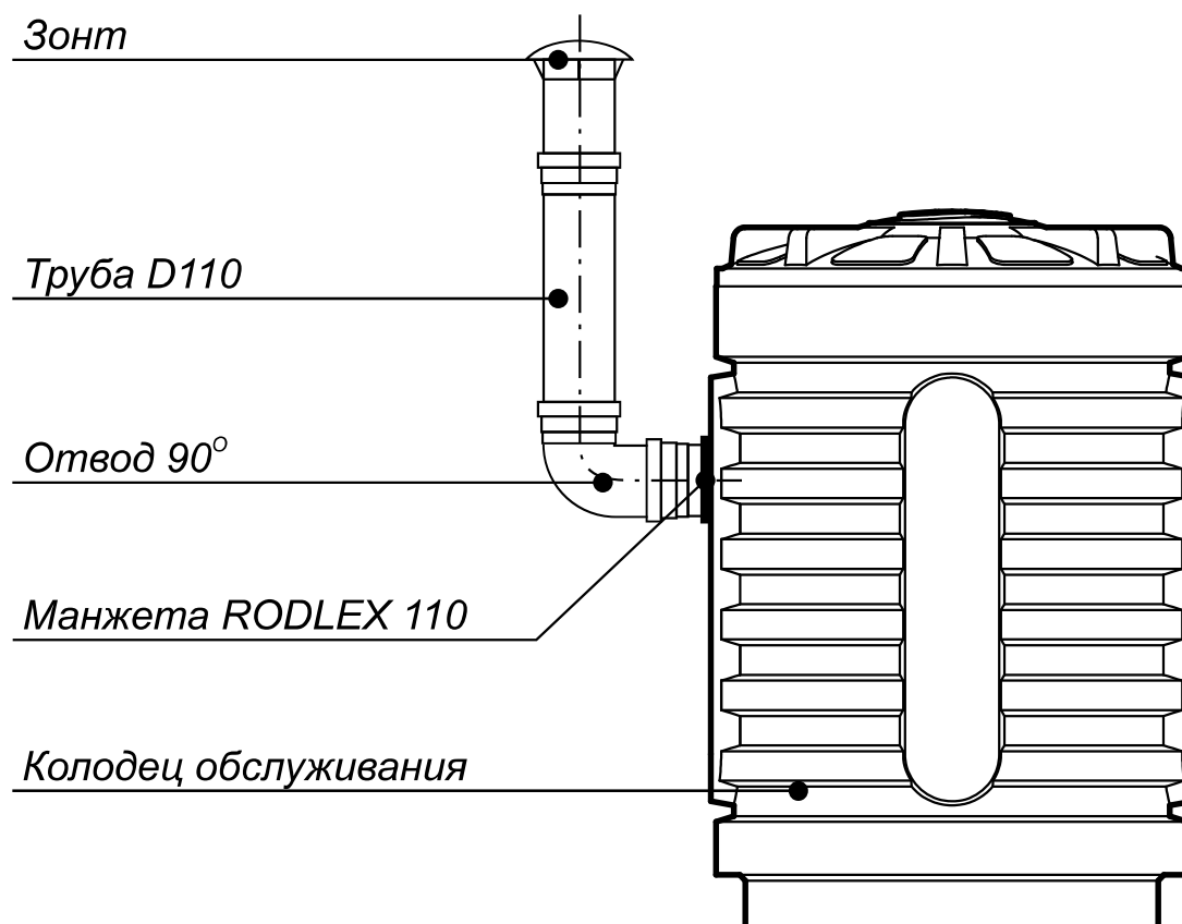
Рис 6. Монтаж технического колодца
