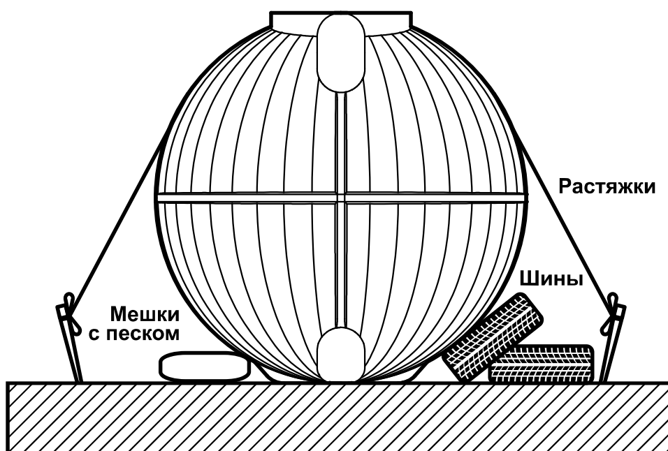
Рис.2 Схема хранения емкости
