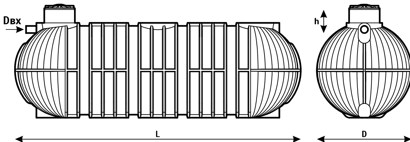
Рисунок 8. Схематичное изображение резервуара.
