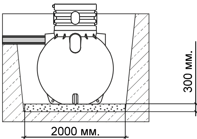
Рисунок 2.2. Схема дренажа
