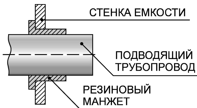
Рисунок 5. Ввод трубопровода
