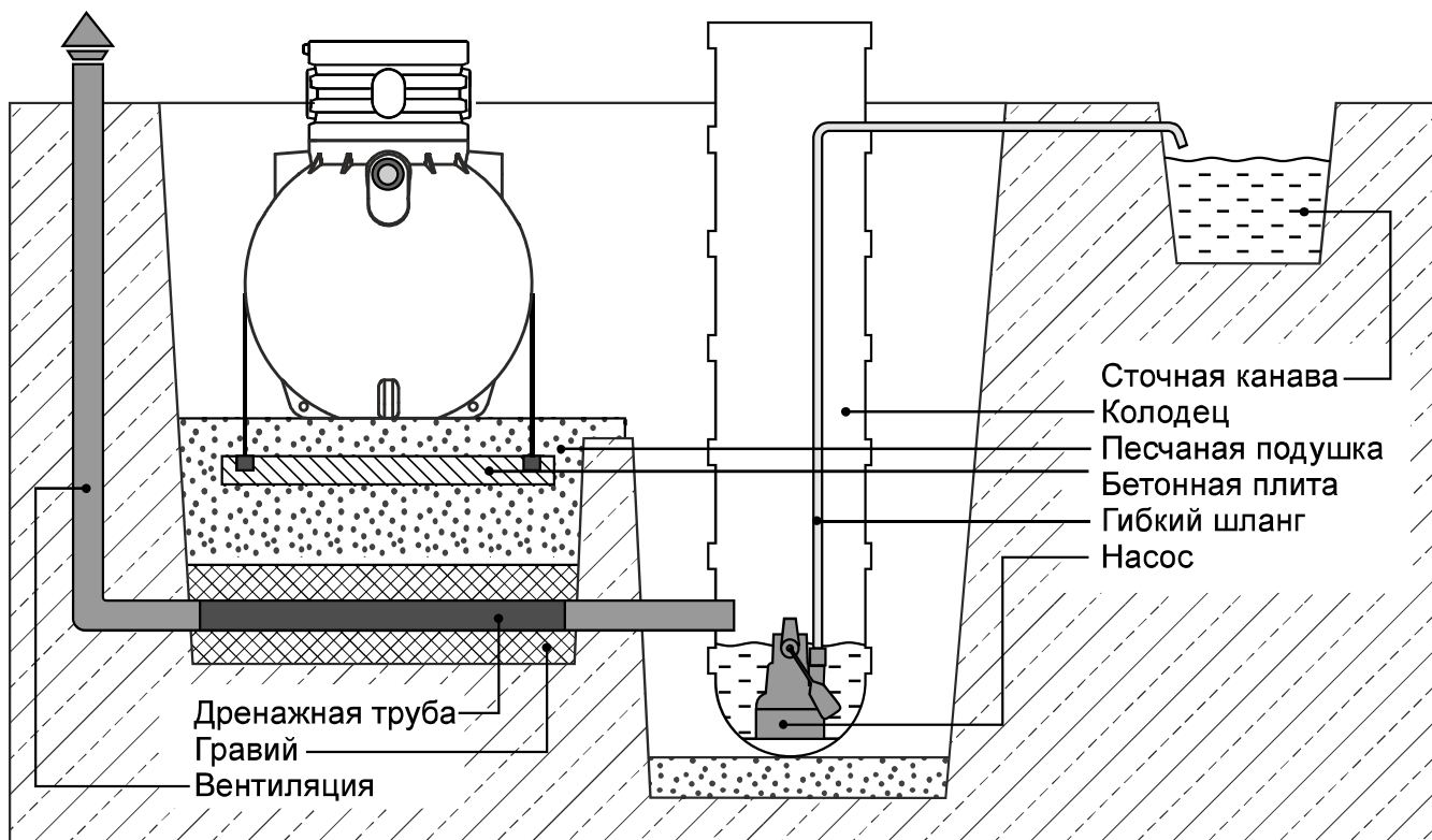
Рисунок 2.2. Схема дренажа
