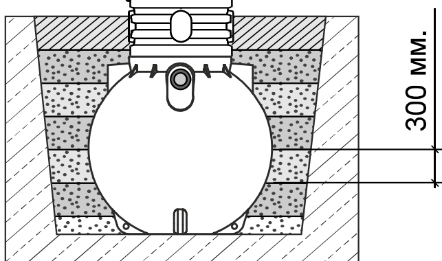
Рисунок 6. Послойная засыпка емкости
