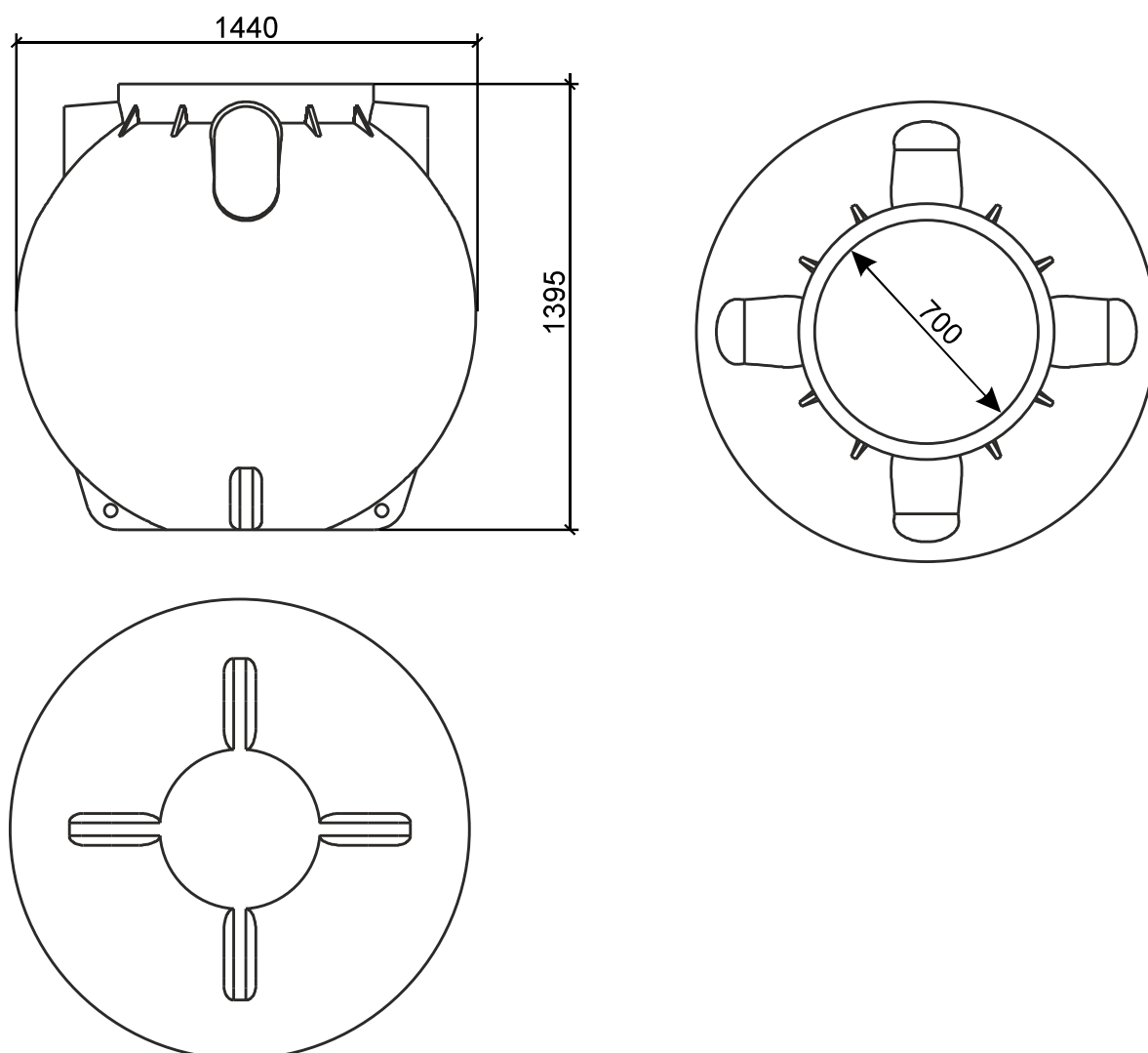
Рисунок 1. Схематичное изображение емкости
