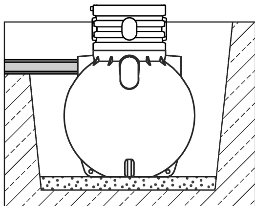
Рисунок 4. Установка емкости
