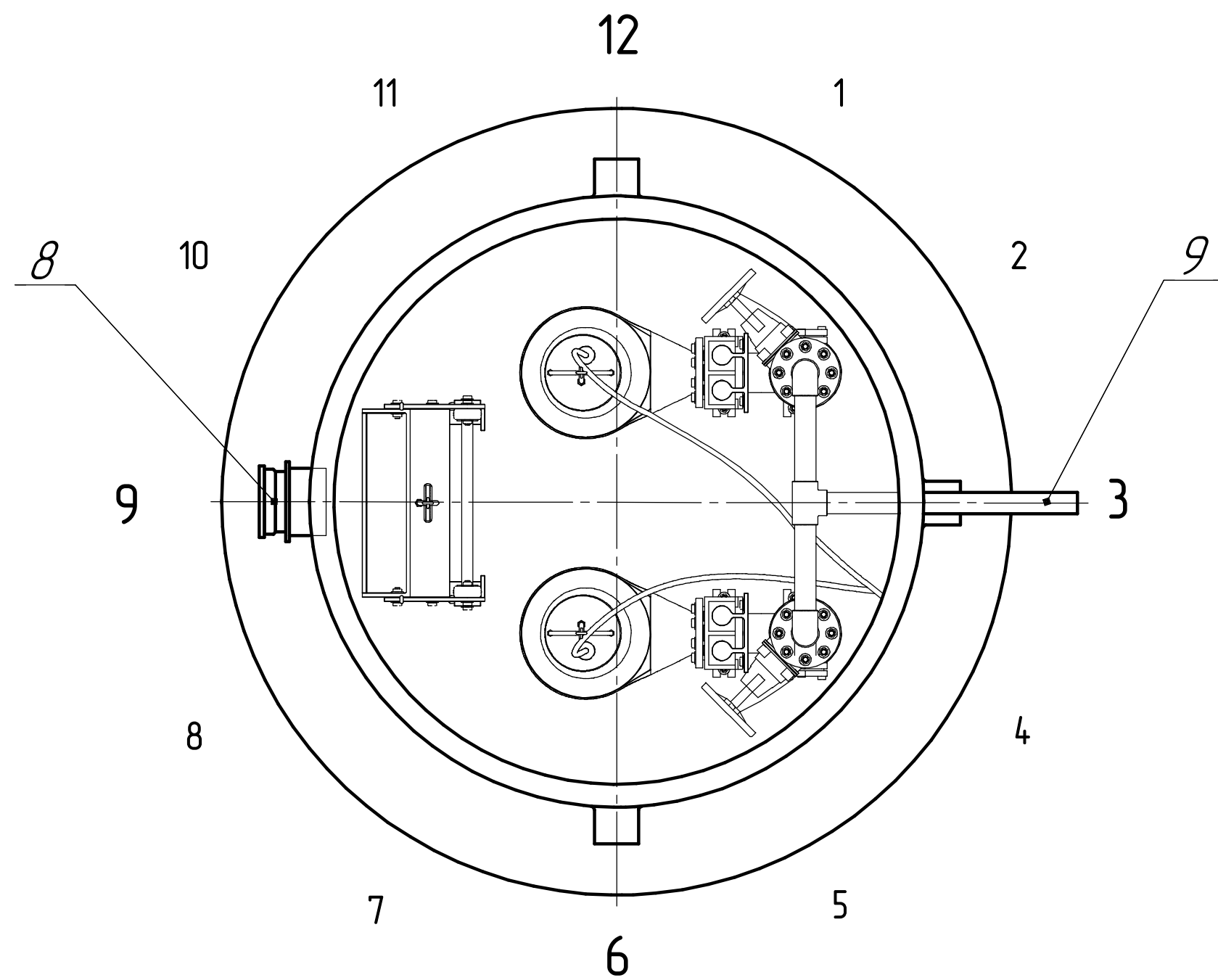
Типы соединений подводящего и напорного патрубка
